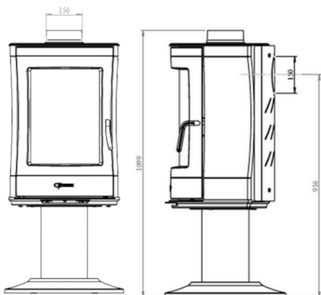
Dimensions : BOMY
